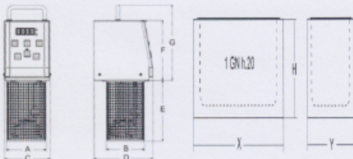
Vasca inox con coperchio opzionale
